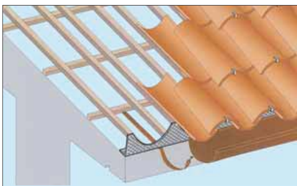
Sistema di posa di coppi di canale privi di dentelli di arresto su doppia orditura di listelli (alla piemontese) con dispositivo di fissaggio meccanico (ganci) sull'elemento di coperta
